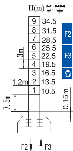
固定式 Stationary
