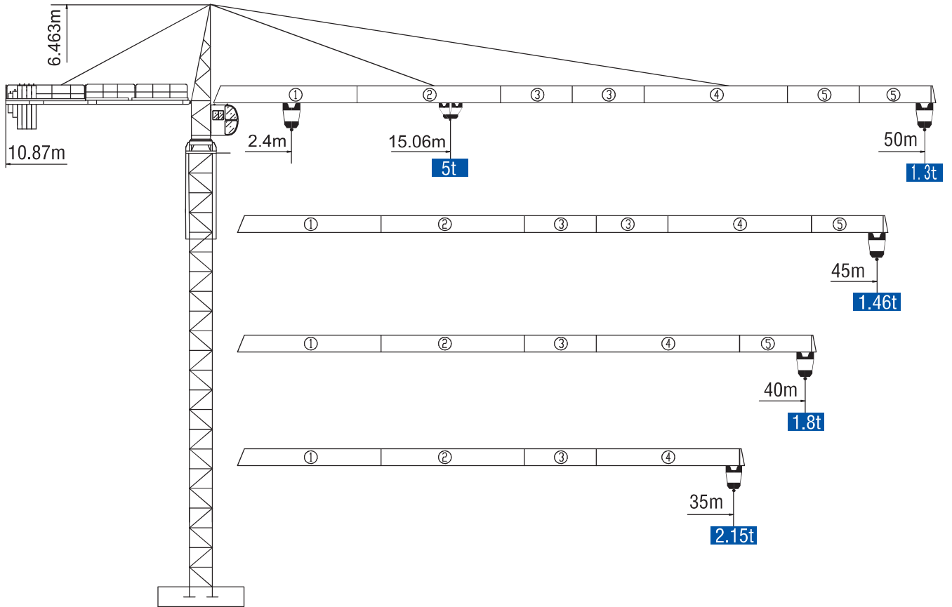
内爬式 Inner-climbing type
