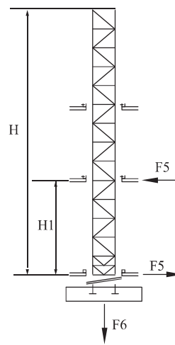
内爬式 Inner-climbing type
