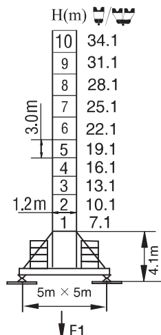
底架压重式 Under frame loading
